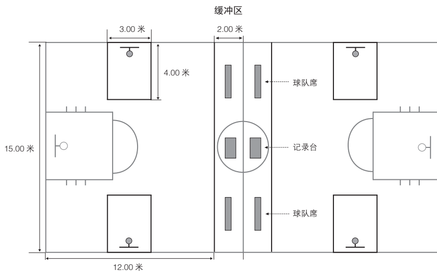
图 36 小篮球四对四比赛场地尺寸图
