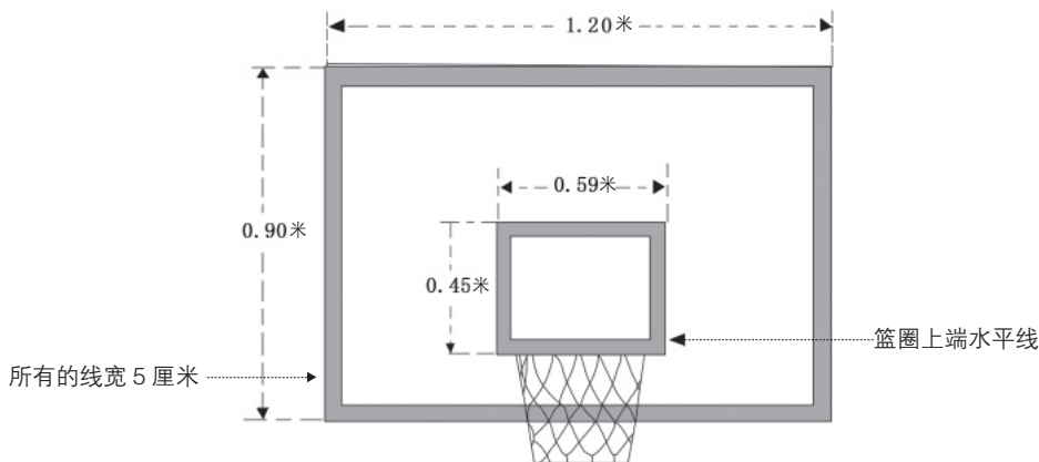
图2 小篮球篮板尺寸图
