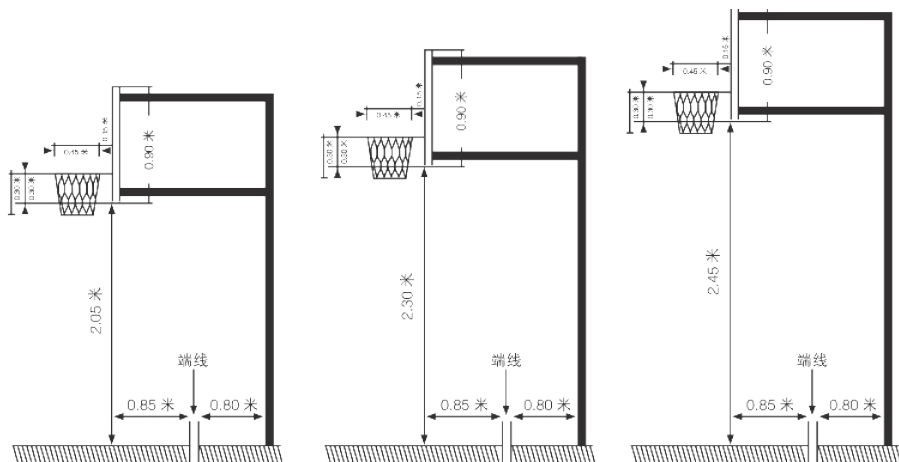
图3 小篮球篮架及球篮尺寸图
